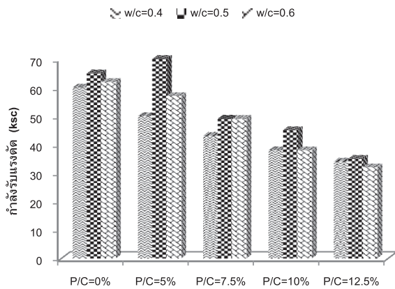
รูปที่ 8 กำลังรับแรงดัดของมอร์ตาร์ผสมน้ำยางพารา
