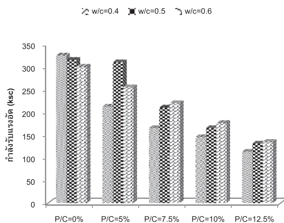
รูปที่ 7 กำลังรับแรงอัดของมอร์ตาร์ผสมน้ำยางพารา
