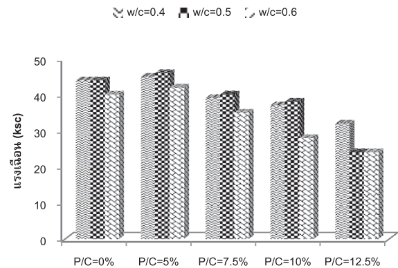
รูปที่ 9 กำลังรับแรงดึงมอร์ตาร์ผสมน้ำยางพารา
