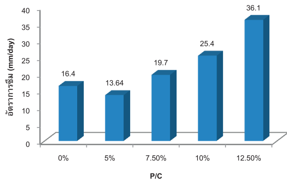
รูปที่ 12 อัตราการรั่วซึมของแบบจำลอง
