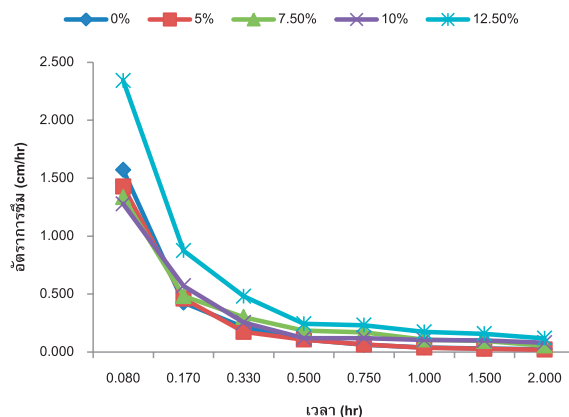
รูปที่ 11 อัตราการรั่วซึมจากสมการของ Horton
