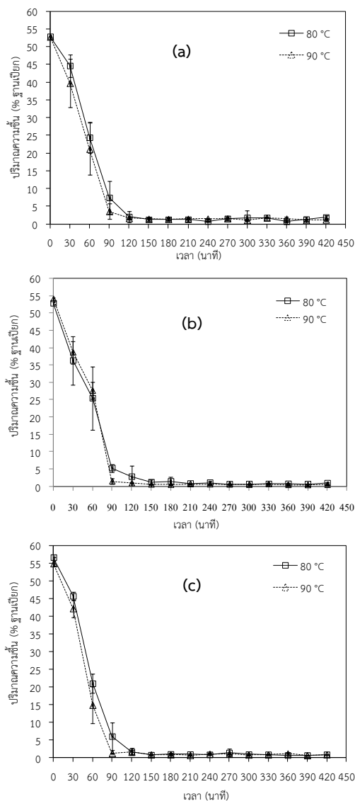
รูปที่ 1 แสดงจลนพลศาสตร์การอบแห้งของเนื้อมะพร้าวชูดที่ผ่านการเตรียมขั้นต้นด้วยวิธีการต่างๆ; ตัวอย่างควบคุม (a), ลวกด้วยไอน้ำ 5 นาที (b) ผสม 1 % โซเดียมเมตาไบซัลไฟต์ (1 กรัม/1 กิโลกรัมตัวอย่าง) (c) ในระหว่างการอบแห้งที่อุณหภูมิ 80 และ 90 องศาเซลเซียส
