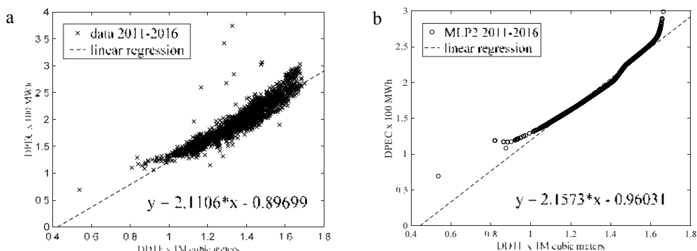
Fig. 4 Long-term EnB : (a) LR; (b) MLP
